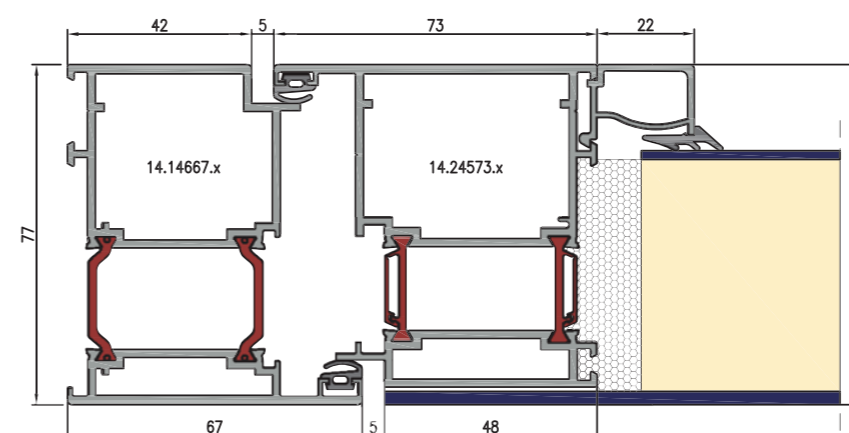
Przekrój przez drzwi panelowe jednostronnie licowane
